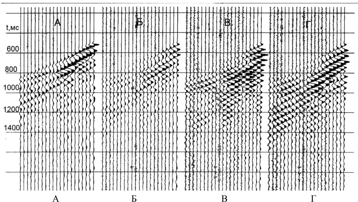
Рис.6. Пример сейсмограмм: А – режим одновременного возбуждения; Б – режим А, но с дополнительной обработкой согласованным фильтром; В – режим последовательного возбуждения с периодом 50 мс и согласованной фильтрацией с периодом 50 мс; Г – режим В, но согласованной фильтрацией с периодом 60 мс.
