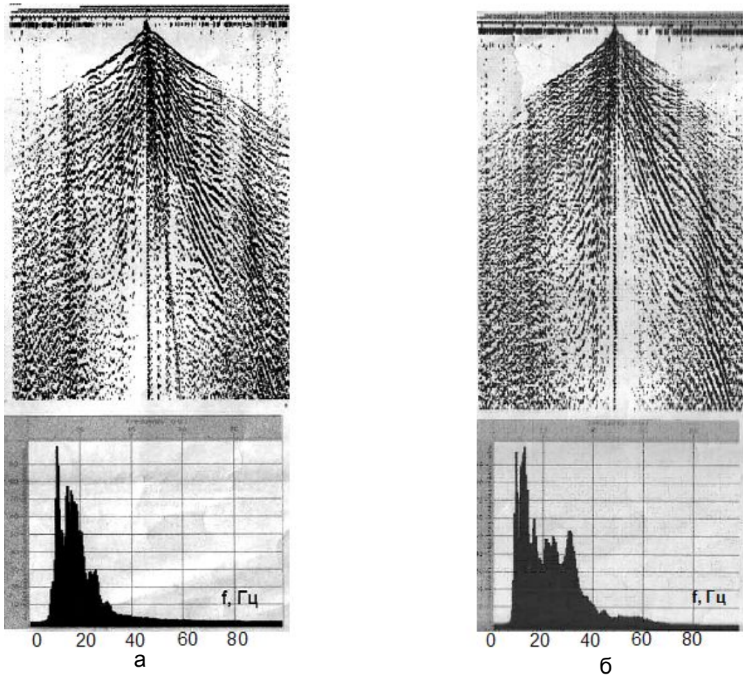
Рис.5. Сейсмограммы и усредненные спектры сигналов, наблюдаемых при работающем (а) и заглушенном (б) двигателе источника
