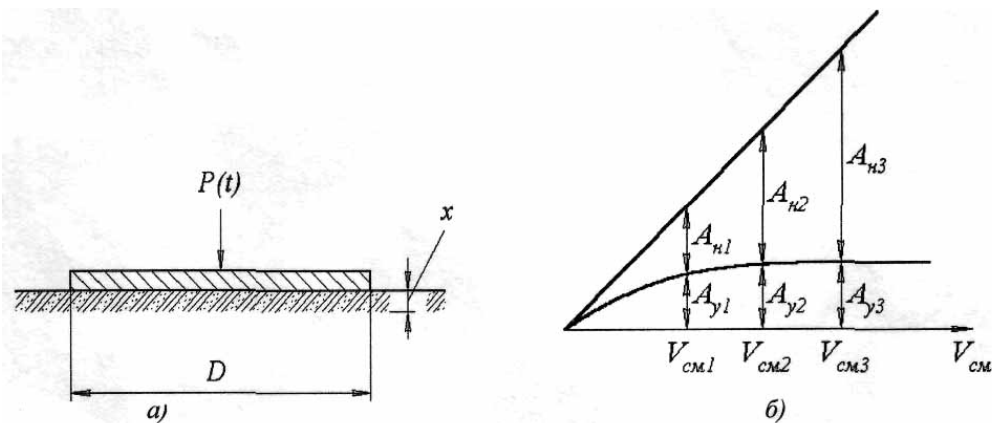
Рис. 1 а)- упрощенная принципиальная схема; б) – качественная зависимость энергии A_n – неупругой и A_v – упругой деформации грунта от скорости смещения V_{см}
